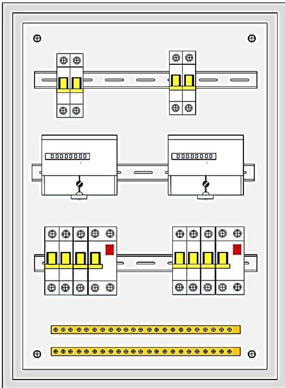
План расположения оборудования в щите
